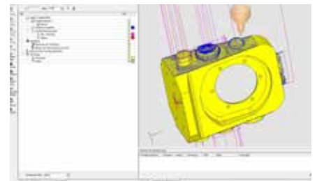
Brandl hat meist sehr genaue Vorstellungen, wie die Maschine ein Werkstück bearbeiten soll (Bild li.). Die Cimatron-Software setzt diese Ideen schnell und präzise um.
