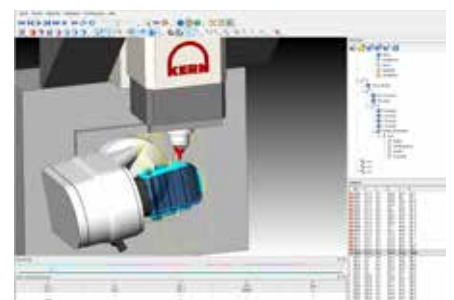
Speziell bei Losgröße 1 ist eine zuverlässige Simulation von großem Vorteil. Bei Cimatron arbeitet dieses Modul mit den Echtzeiten aus dem Postprozessor.
